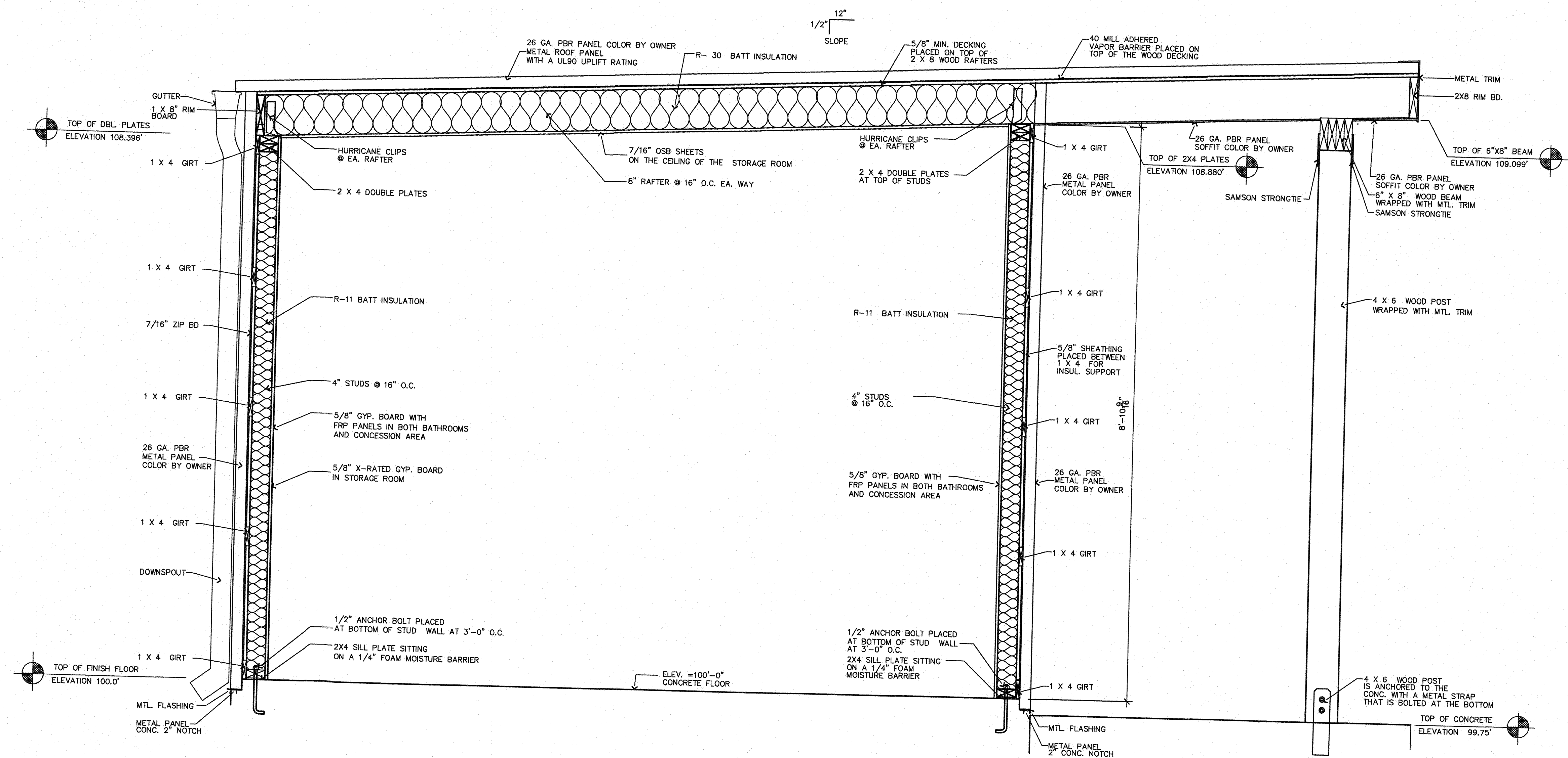
A WALL SECTION (TYP.) SCALE: 1" = 1'-0"
